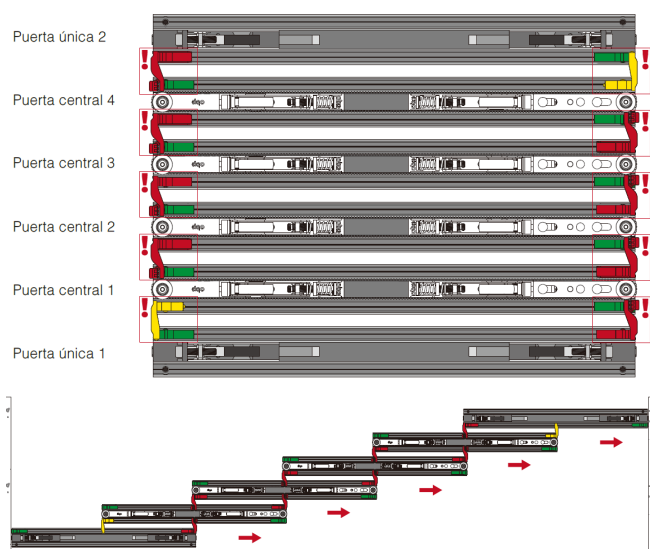
APERTURA HACIA LA DERECHA (VISTA DESDE ABAJO)
