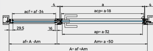
Versión con fijo lateral
