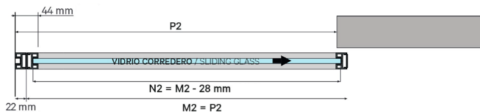
PLANTA CON PERFIL RECEPTOR
