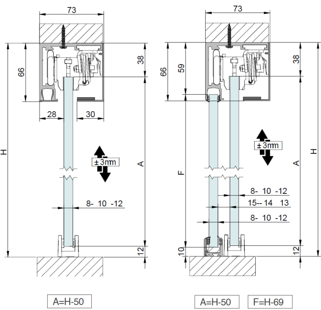
MONTAJE A TECHO
