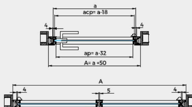
2P - Solo versión cierre magnético
