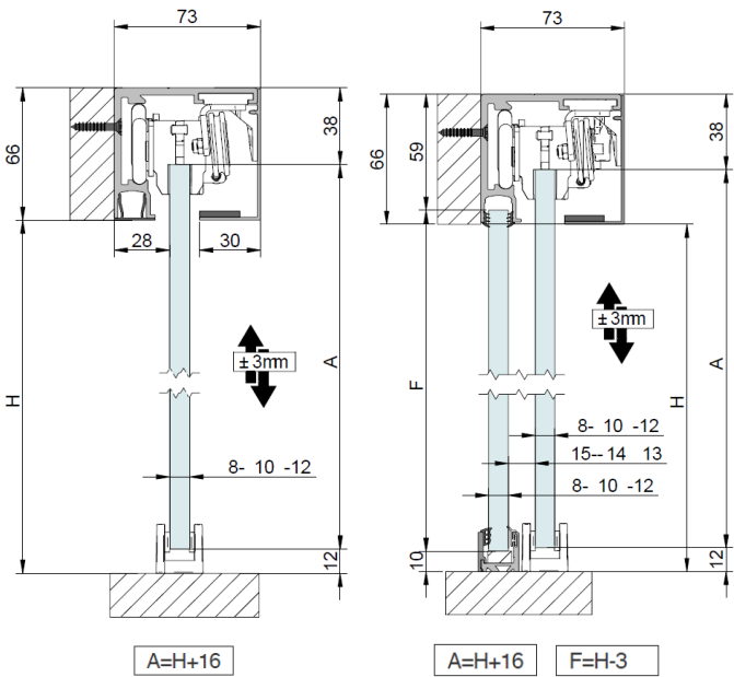
MONTAJE A PARED
