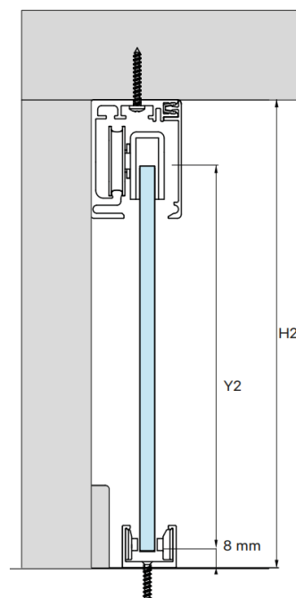
PERFIL A TECHO
