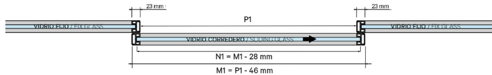
PLANTA SIN PERFIL RECEPTOR (FRAME FRONT)
