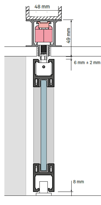
PERFIL EMPOTRADO "T"
